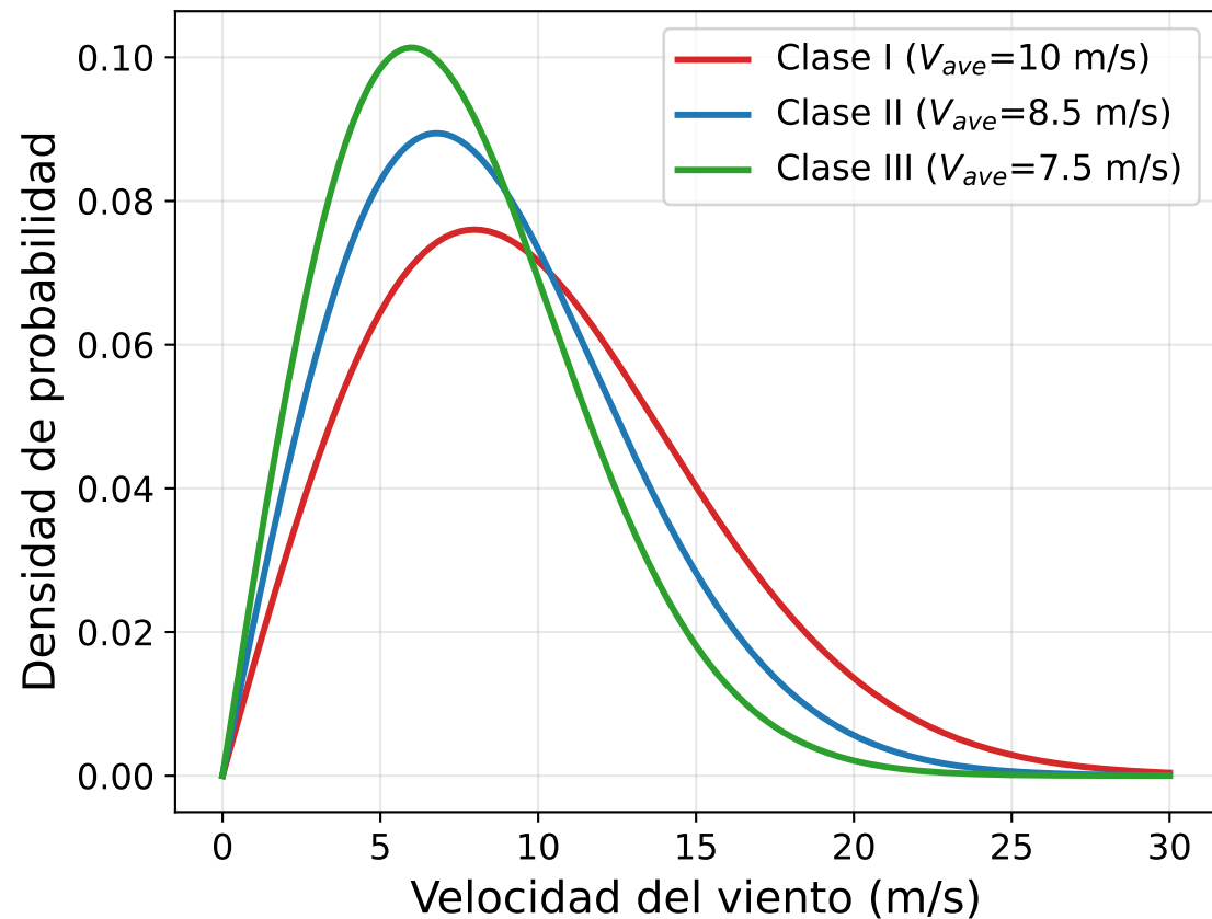
(a) Efecto de c : clases IEC ( k = 2 )
