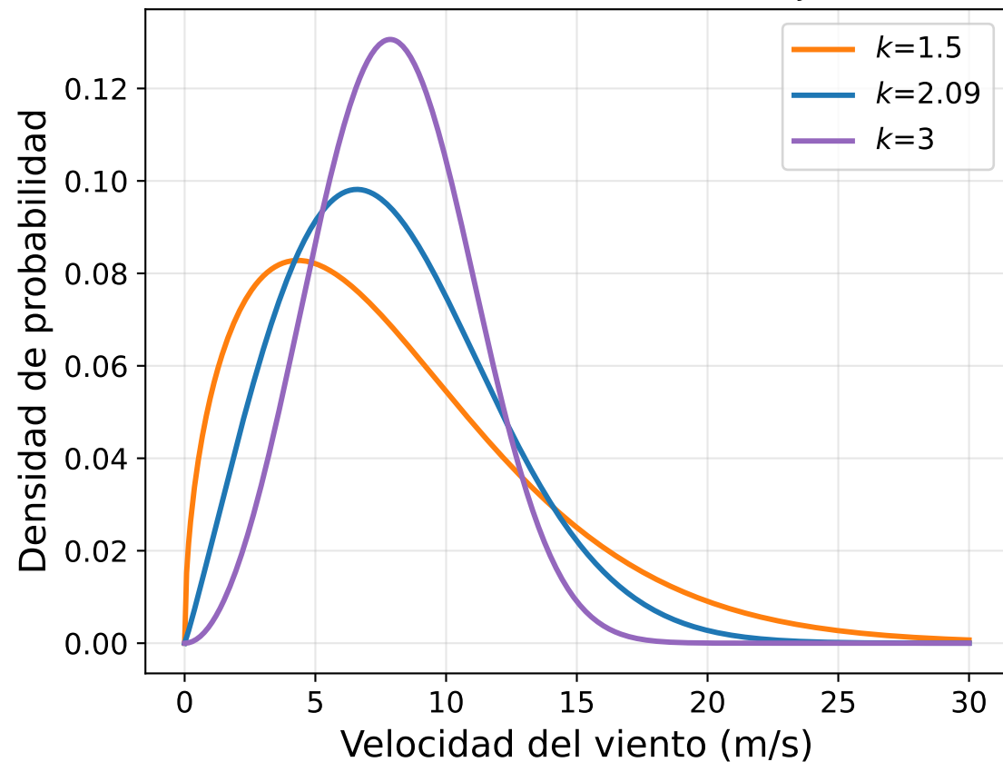
(b) Efecto de k : c=9 m/s fijo
